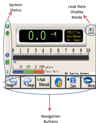
Interfaz gráfica de usuario táctil
